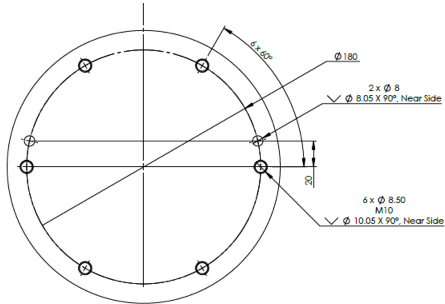
1.1: 機器人底座的底部視圖
